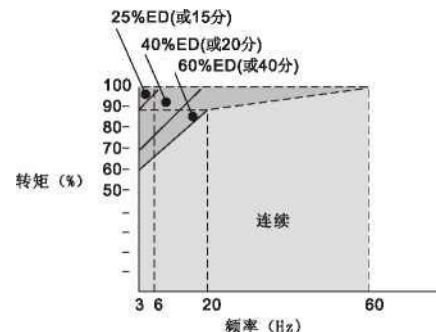
本公司标准电机的容许负载特性
