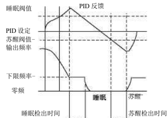
F08.12=1 示意图（睡眠方式 1）
