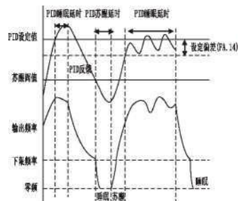
F08.12=2 示意图（睡眠方式 2）
