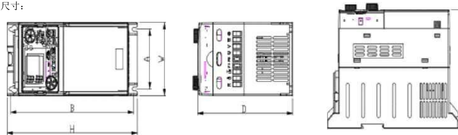
图 D-1 变频器 0.75KW~110KW 尺寸
